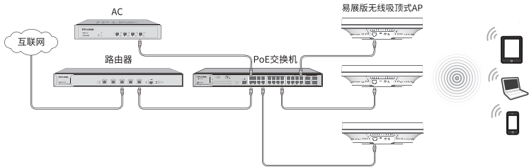
图4-7 典型应用拓朴图-有线组网
